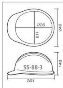
SS-88-3 型寸法図
