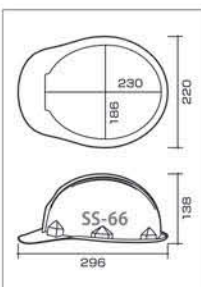
SS-66 型寸法図
