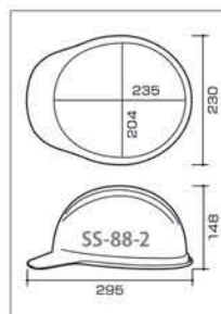
SS-88-2 型寸法図
