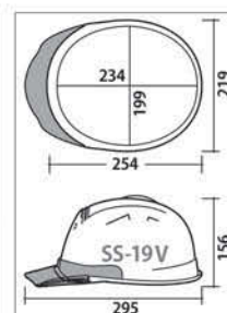
寸法図
