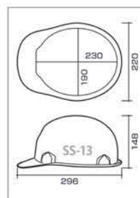
SS-13 型寸法図
