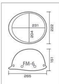
FM-6 型寸法図
