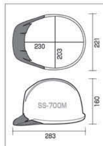
SS-700M 型寸法図
