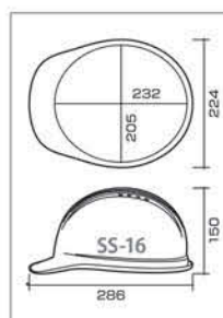
SS-16V 型寸法図
