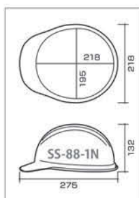
SS-88-1N 型寸法図
