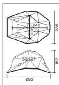
SS-21 型寸法図
