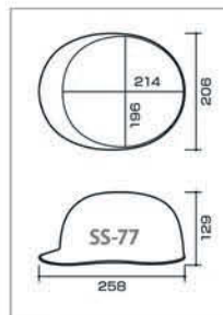
SS-77 型寸法図
