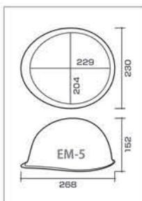
EM-5 型寸法図
