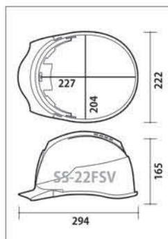
寸法図
