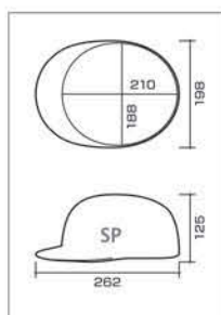
SP 型寸法図
