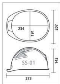
SS-01 型寸法図
