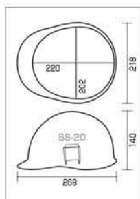
SS-20 型寸法図
