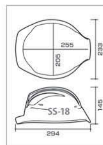
SS-18V 型寸法図
