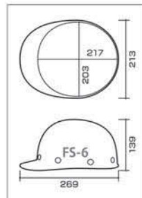
FS-6 型寸法図
