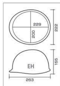
EH 型寸法図
