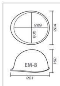
EM-8 型寸法図
