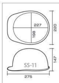
SS-11 型寸法図
