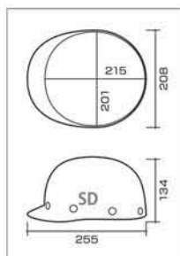
SD 型寸法図
