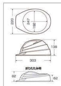
IZANO 寸法図
