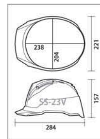
SS-23V 寸法図
