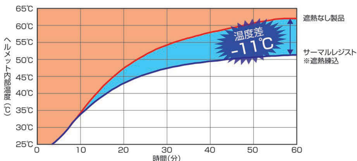
遮熱性能比較実験(当社試験)
