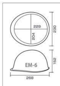
EM-6 型寸法図
