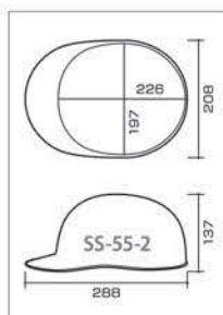
SS-55-2 型寸法図
