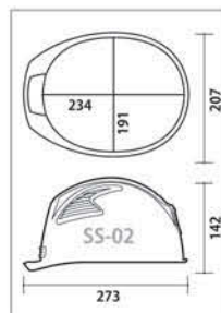
SS-02 型寸法図
