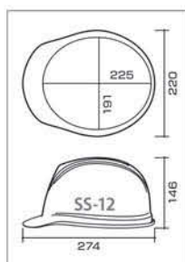
SS-12 型寸法図
