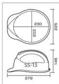
SS-15 型寸法図
