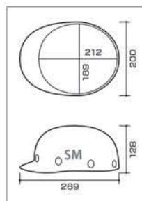
SM 型寸法図
