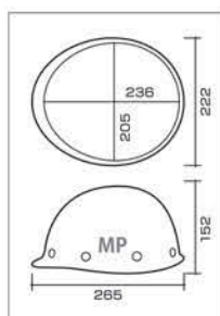
MP 型寸法図
